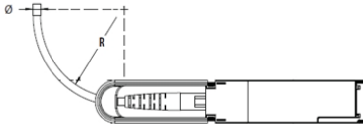
图4-36 AOC 光缆弯曲半径示意图
