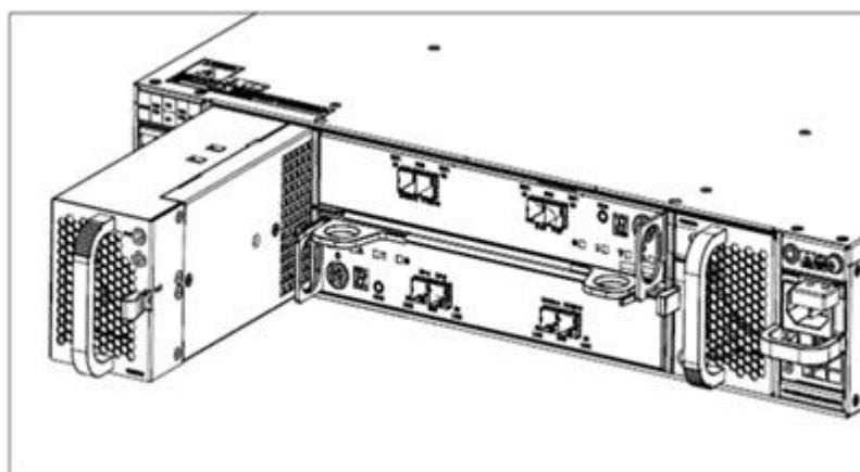
图4-18 安装 SSU2225B 风扇模块+电池模块示意图
