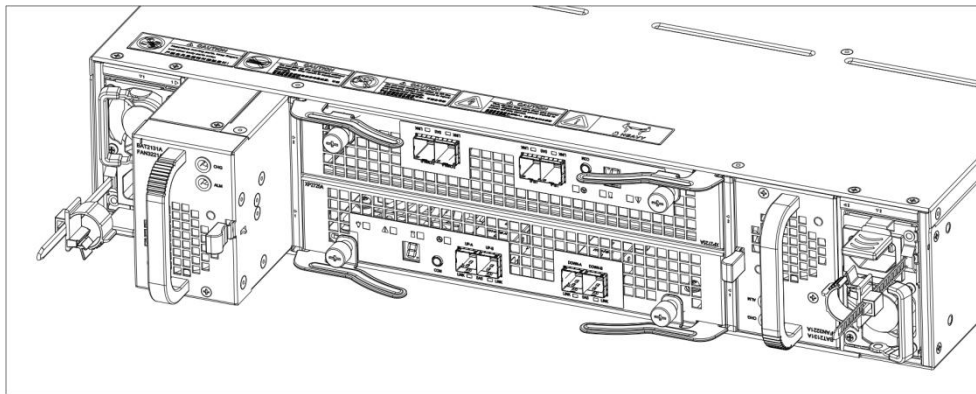
图6-9 安装/拆卸 SSU2725B 风扇模块+电池模块示意图
