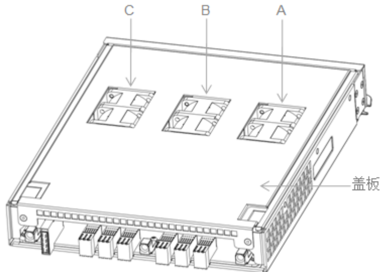
图6-11 SSU2725B/SSU2725 内置风扇模块安装位置示意图
