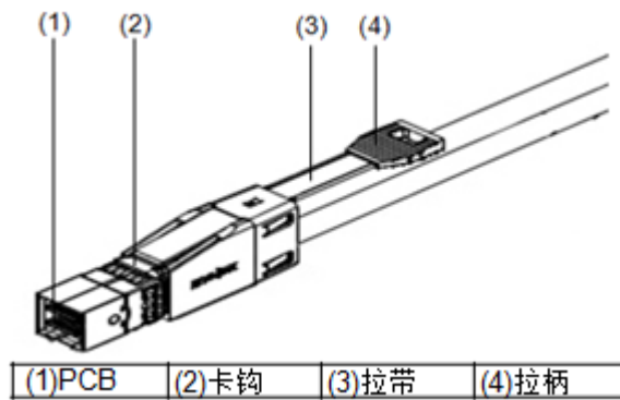
图4-34 SAS 线缆上 Mini SAS HD 连接器示意图
