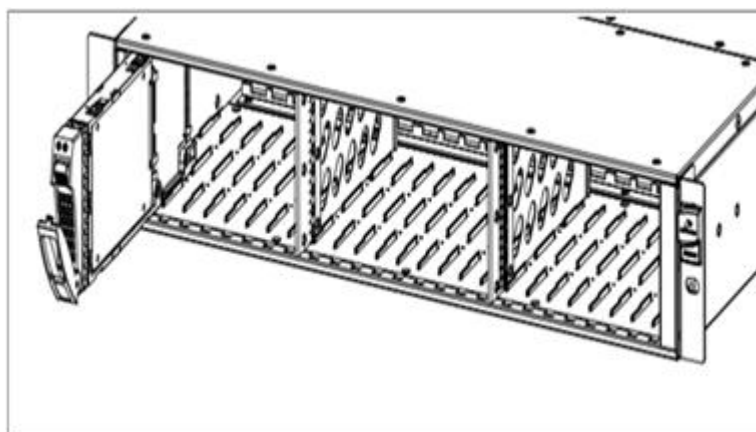
图6-18 安装 2.5 英寸磁盘模块 A 示意图（二）
