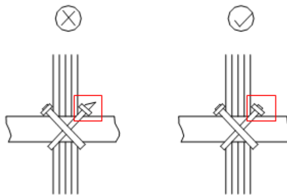
图4-22 线缆捆扎示意图（二）
