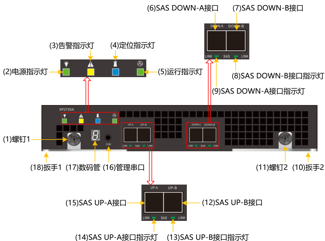
图3-18 SSU2725B/SSU2725 的 XP 正视图
