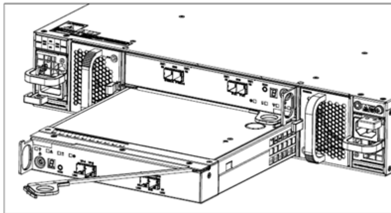
图6-6 安装/拆卸 SSU2225 XP 示意图
