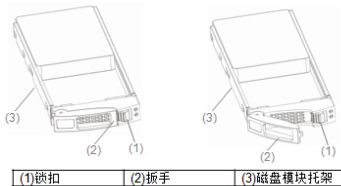
图6-19 2.5 英寸磁盘模块 B 示意图
