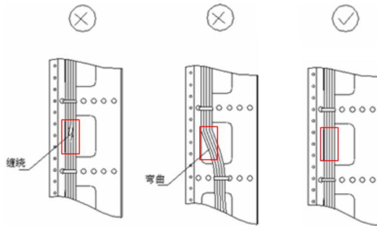
图4-21 线缆捆扎示意图（一）
