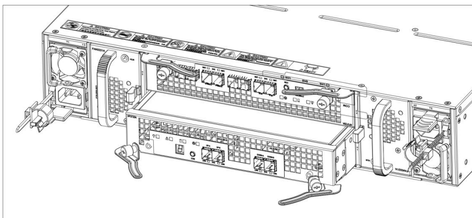
图6-7 安装/拆卸 SSU2725 XP 示意图
