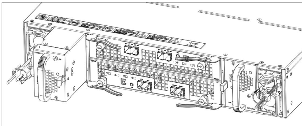
图6-13 安装/拆卸 SSU2725 后端风扇模块示意图
