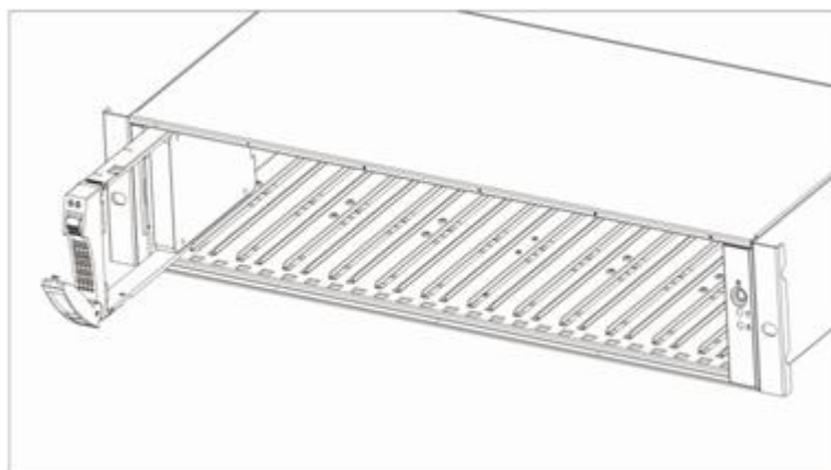
图6-22 安装 2.5 英寸磁盘模块 B 示意图（二）
