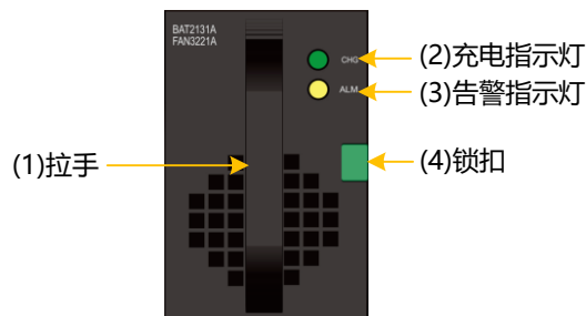
图3-19 SSU2725B 风扇模块+电池模块正视图
