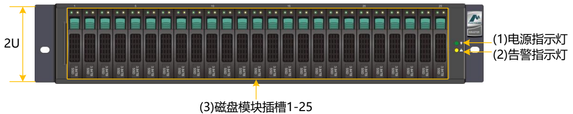
图3-15 SSU2725B/SSU2725 前正视图
