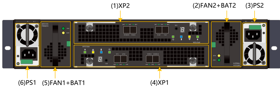
图3-16 SSU2725B 后正视图
