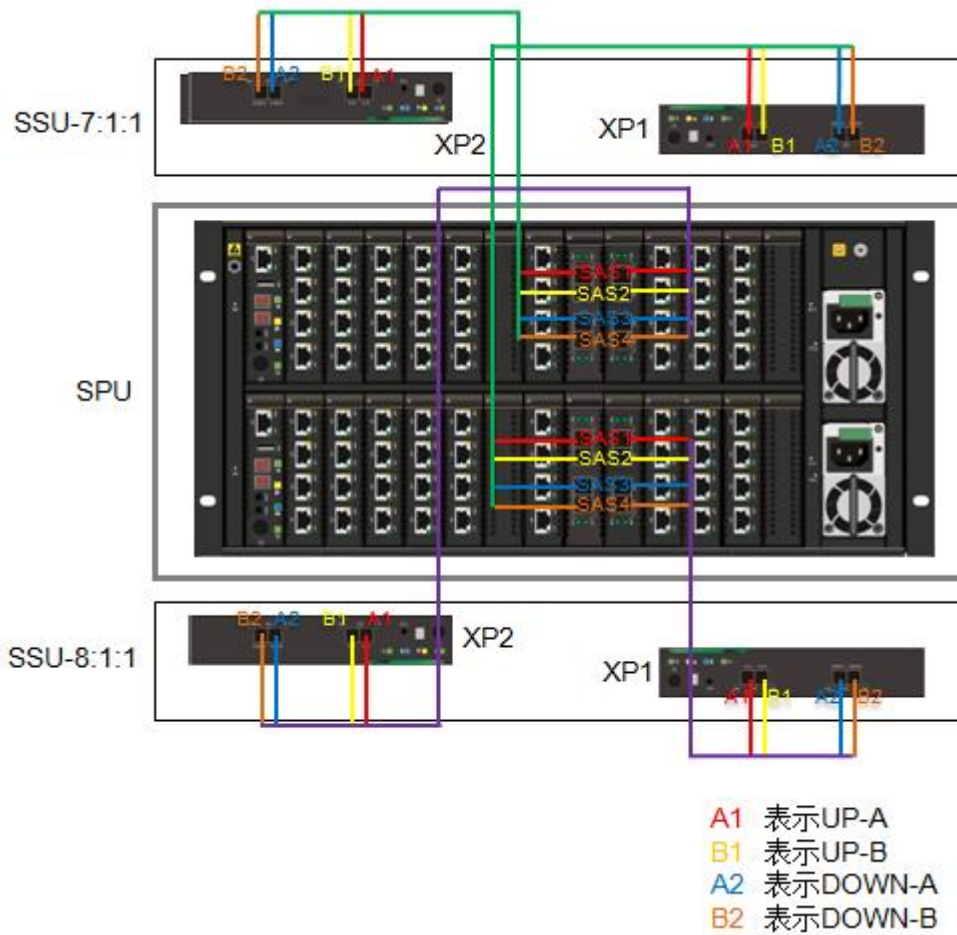
图4-37 SAS 线缆安装示意图
