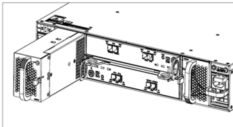
图6-10 安装/拆卸 SSU2225 风扇模块示意图
