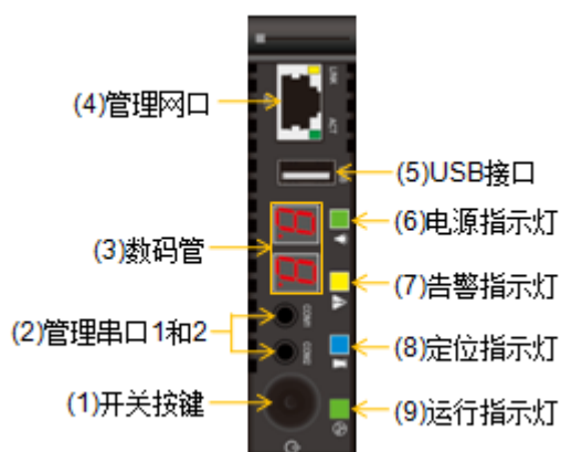
图3-4 SP 管理插卡正视图
