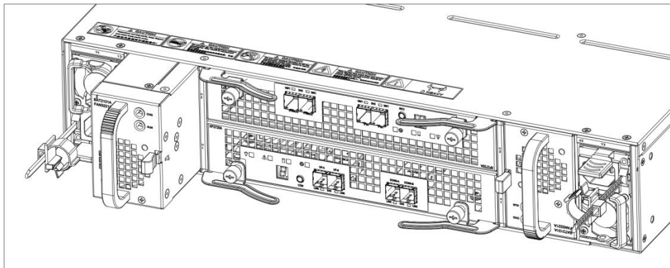
图4-19 安装 SSU2725B 风扇模块+电池模块示意图
