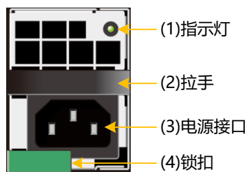
图3-14 SSU2225B/SSU2225 电源模块正视图
