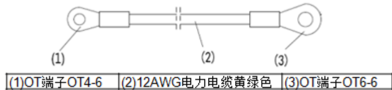
图4-25 接地线示意图
