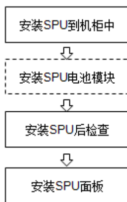
图4-12 SPU 安装流程示意图
