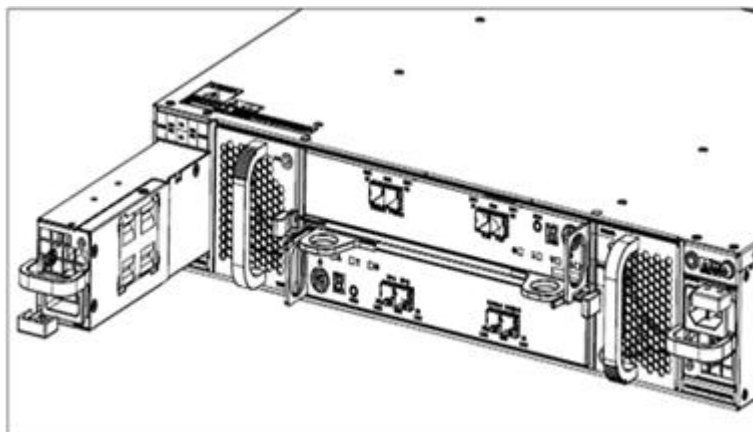
图6-14 安装/拆卸 SSU2225 电源模块示意图
