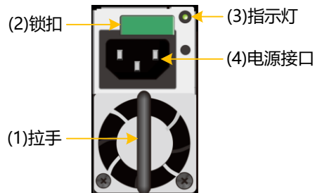
图3-23 SSU2725 电源模块正视图
