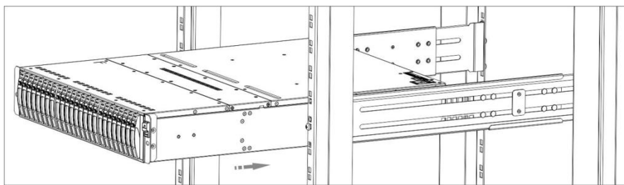
图4-17 安装 SSU 示意图
