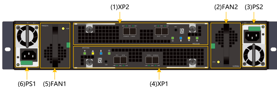
图3-17 SSU2725 后正视图
