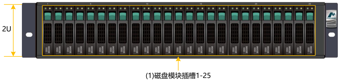
图3-8 SSU2225B/SSU2225 前正视图
