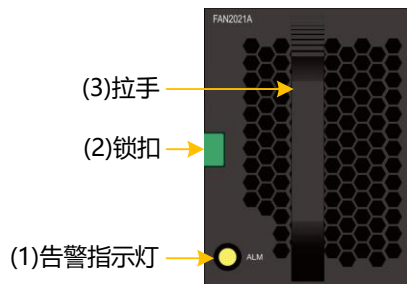
图3-13 SSU2225 风扇模块正视图
