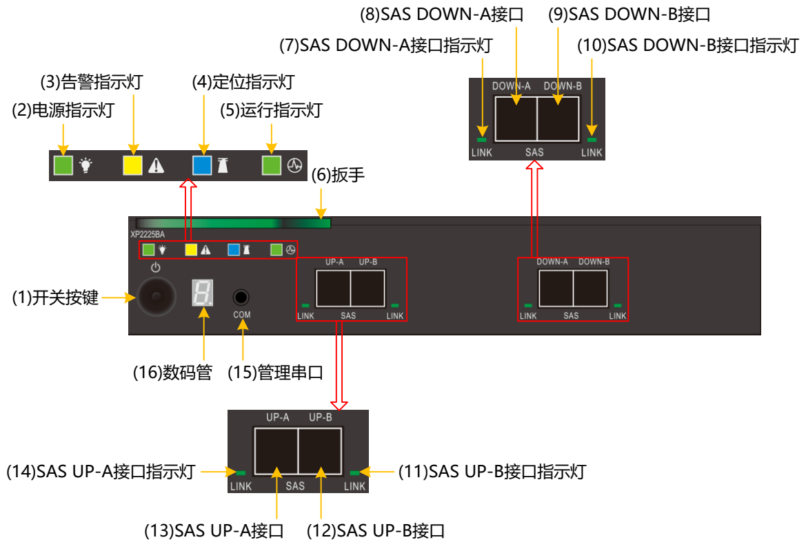
图3-11 SSU2225B/SSU2225 的 XP 正视图
