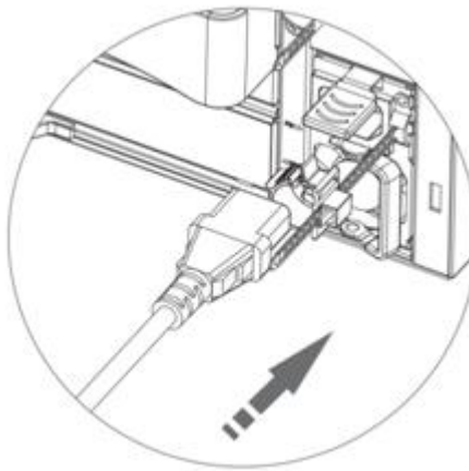
图4-31 安装电源线示意图（三）
