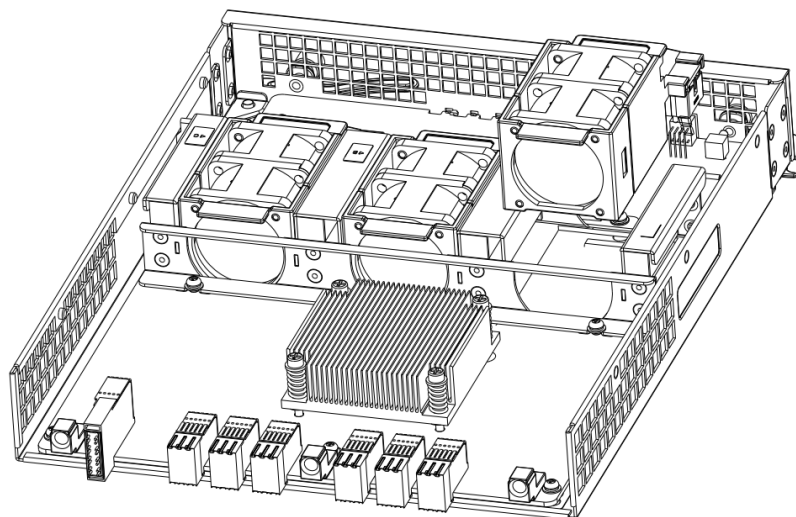
图6-12 安装/拆卸 SSU2725B/SSU2725 内置风扇模块示意图
