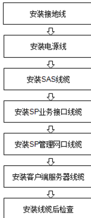
图4-24 线缆安装流程示意图
